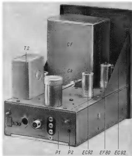
Bild 4. Der Aufbau und die Rückansicht des Meßsenders und Frequenzmessers. Das Bild läßt die Abschirmungen des Dreh- und Korrekturkondensators (Cf + Ck) sowie des Hf-Spannungsteilers P 1 gut erkennen
