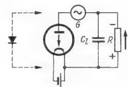
Bild 8.2. Einweg-Gleichrichtung mit Gleichrichterröhre (daneben Ersatzmöglichkeit der Röhre durch einen „Trockengleichrichter“)
