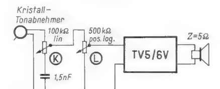
Bild 4. Anordnung eines Klangeinstellers K und eines Lautstärkeeinstellers L
