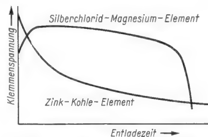
Bild 1. Typische Entladungskurven von Silberchlorid-Magnesium-Zellen und Zink-Kohle-Elementen
