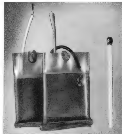
Bild 2. Zweizellige Silberchlorid-Magnesium-Batterie für den Modellbau
