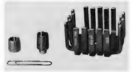
Kühlkörper für Hochleistungs-Transistoren in verschiedenen Bauformen. Der fingerartige Aufbau des rechten Modells gibt die Wärme besonders gut an die Luft ab
