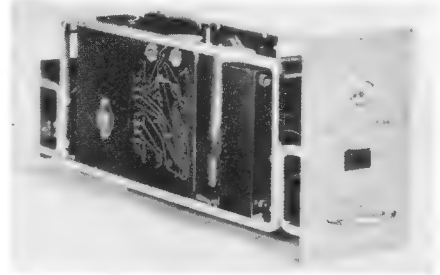
Einschubausführung des Konstantspannungsgerätes PE 4863; links neben der gedruckten Schaltung sieht man auf der Kühlplatte einen Leistungstransistor
