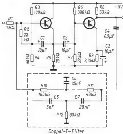
Bild 3. Schaltung eines Transistor-Verstärkers mit frequenzabhängiger Gegenkopplung durch ein Doppel-T-Filter
