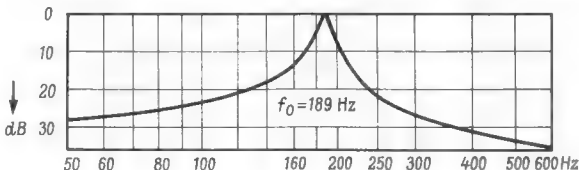
Bild 5. Dämpfungskurve eines auf 189 Hz abgestimmten Doppel-T-Filters über den Frequenzbereich 50 bis 600 Hz
