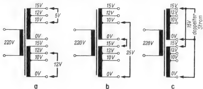
Schaltbeispiele für die Elektronik-Netztransformatoren; a = zwei einzelne Spannungen, b = höhere Spannung durch Serienschaltung, c = doppelter Strom durch Parallelschaltung
