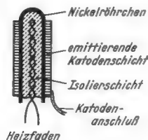
Bild 8.5. Schnitt durch eine indirekt geheizte Katode
