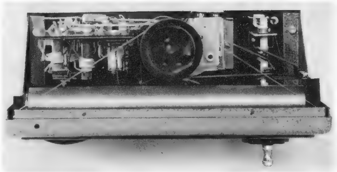
Bild 7. Aufsicht auf das Chassis
