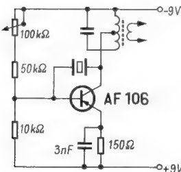
Bild 5. Oszillator für Obertonquarze 15 MHz bis 100 MHz
