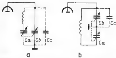
Bild 3. Wirkungsweise des Schwingkreises L 3'. Der Plattensatz Ca liegt elektrisch mit Cb in Serie, Cc (= Röhren- und Schaltkapazität) mit Cb parallel. Bild 3b ist die gleiche Schaltung wie Bild 3a, es ist nur zur besseren Verständlichkeit umgezeichnet
