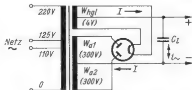
Bild 8.4. Doppelweg-Gleichrichtung mit Gleichrichterröhre
