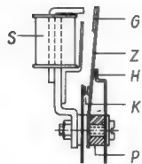
Links: Bild 1. Schematische Darstellung eines Resonanzrelais
