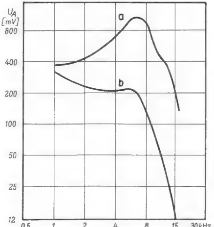
Bild 5. Frequenzgang bei hohen Frequenzen bei Benutzung des Klangeinstellers K aus Bild 4; a = Schleifer des Potentiometers am Tonabnehmer, Höhen angehoben; b = Schleifer am 1,5-nF-Kondensator, Höhen abgesenkt
