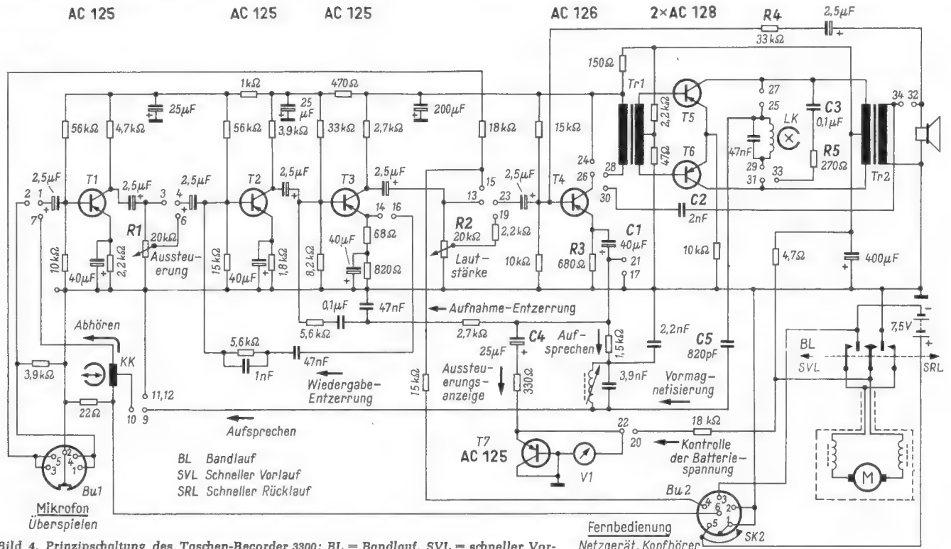
Bild 4. Prinzipschaltung des Taschen-Recorder 3300; BL = Bandlauf, SVL = schneller Vorlauf, SRL = schneller Rücklauf; Stellung der übrigen Schalterkontakte siehe Text
