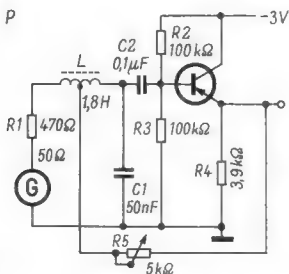
Rechts: Bild 2. Schaltung eines LC-Selektivverstärkers mit Rückkopplung
