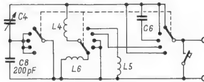
Bild 10. Erweiterter Meßkreis
