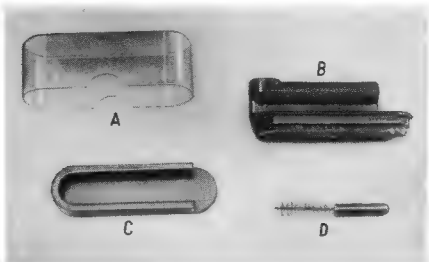
Bild 1. Rexon-Handreiniger für Schallplatten; A = Schutzkappe, B = Reinigungsbürste, C = Sockel zum Schutz der Bürstenfläche bei Nichtgebrauch, D = Bürstchen zum Aufrauhen der Reinigungsfläche
