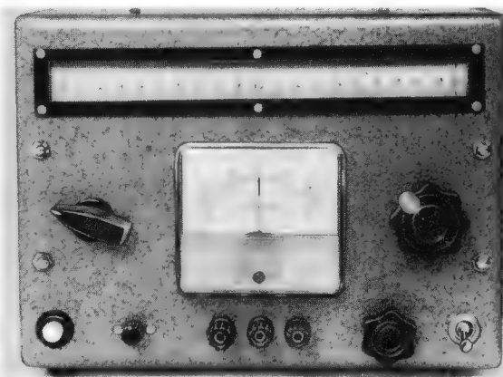
Bild 8. Die Frontansicht des Gerätes mit der provisorischen Eichskala. Das Mikroampere-meter ist ein japanisches Erzeugnis
