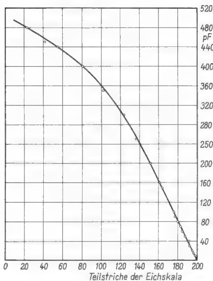
Bild 9. Beispiel einer Eichkurve für den Bereich 1. Zum Eichern wurden lediglich handelsübliche Kondensatoren entsprechend dem aufgedruckten Kapazitätswert verwendet. Wie die Eichpunkte zeigen, sind die Toleranzen erfreulich gering
