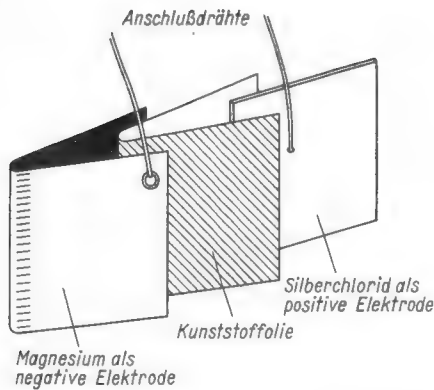
Bild 3. Aufbau einer der in Bild 2 gezeigten Zellen
