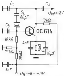
Bild 4. Oszillator für Grundwellenquarze bis 30 MHz
