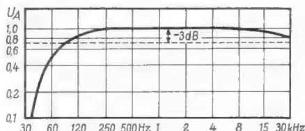
Bild 3. Frequenzgang gemessen an einem 5-Ω-Abschlußwiderstand bei konstanter Eingangsspannung von 50 mV
