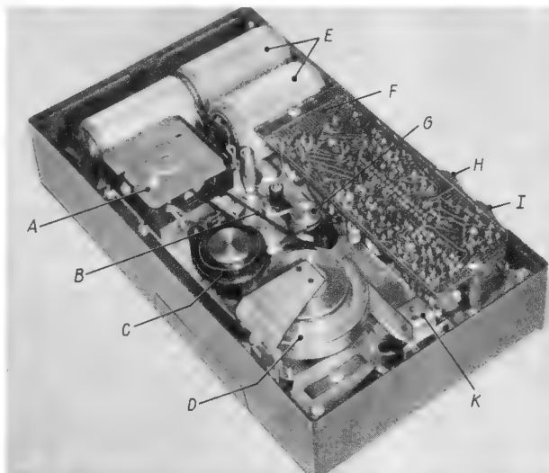
Bild 1. Klein, leicht und vielseitig ist der Philips-Taschen-Recorder 3300; die neu entwickelte Tonbandkassette kann mit einem Griff ausgewechselt werden
