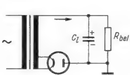
Bild 8.3. Einweg-Gleichrichtung mit Heizung der Gleichrichterröhre aus dem Netztransformator
