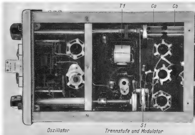
Bild 5. Blick in die Verdrahtung; der Oszillator ist von der Trennstufe und dem Modulator durch eine Abschirmung getrennt
