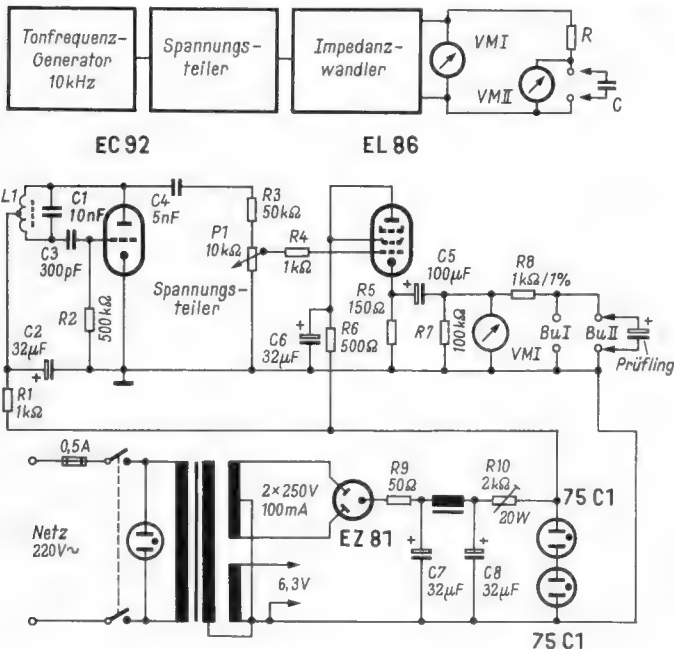
Bild 3. Die Schaltung der Anordnung zum Messen des Scheinwiderstandes von Elektrolytkondensatoren
