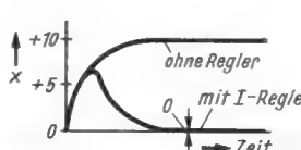
Bild 14. Zeitliches Verhalten des Integralreglers
