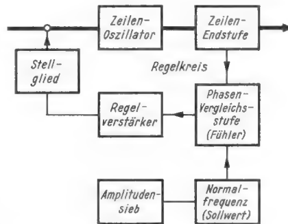
Bild 7. Regelkreis für die Phasensynchronisierung mit Vergleichsstufe und Sollwertgeber
