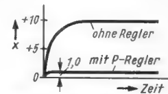
Bild 12. Zeitliches Verhalten des Proportionalreglers
