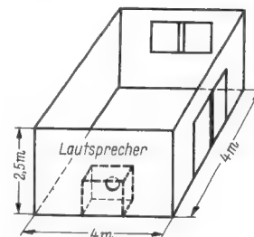
Abmessungen des Wohnraums, die den Berechnungen zugrunde gelegt wurden
